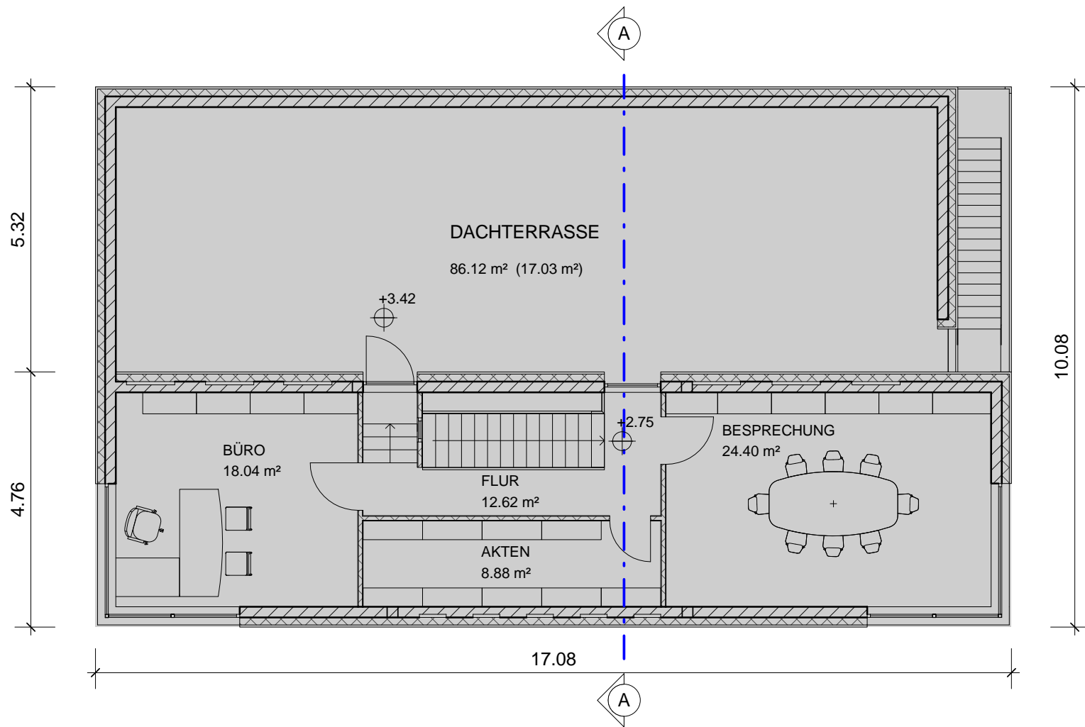
GRUNDRISS OBERGESCHOSS (Gesamtfläche EG 87.29 m 2 )
