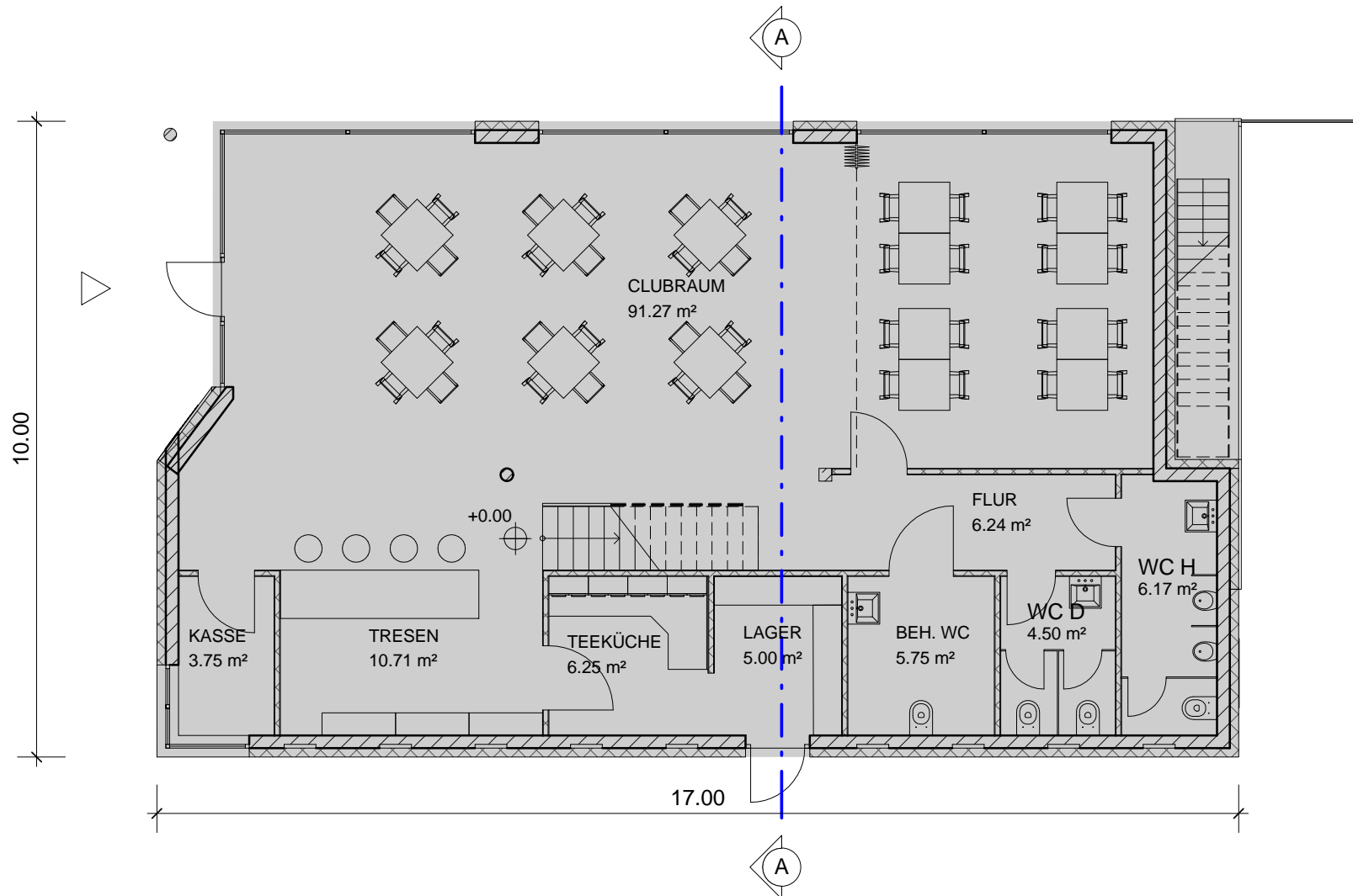
GRUNDRISS ERDGESCHOSS (Gesamtfläche EG 149.47 m²)
